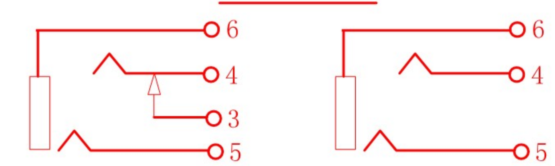
电路原理图
