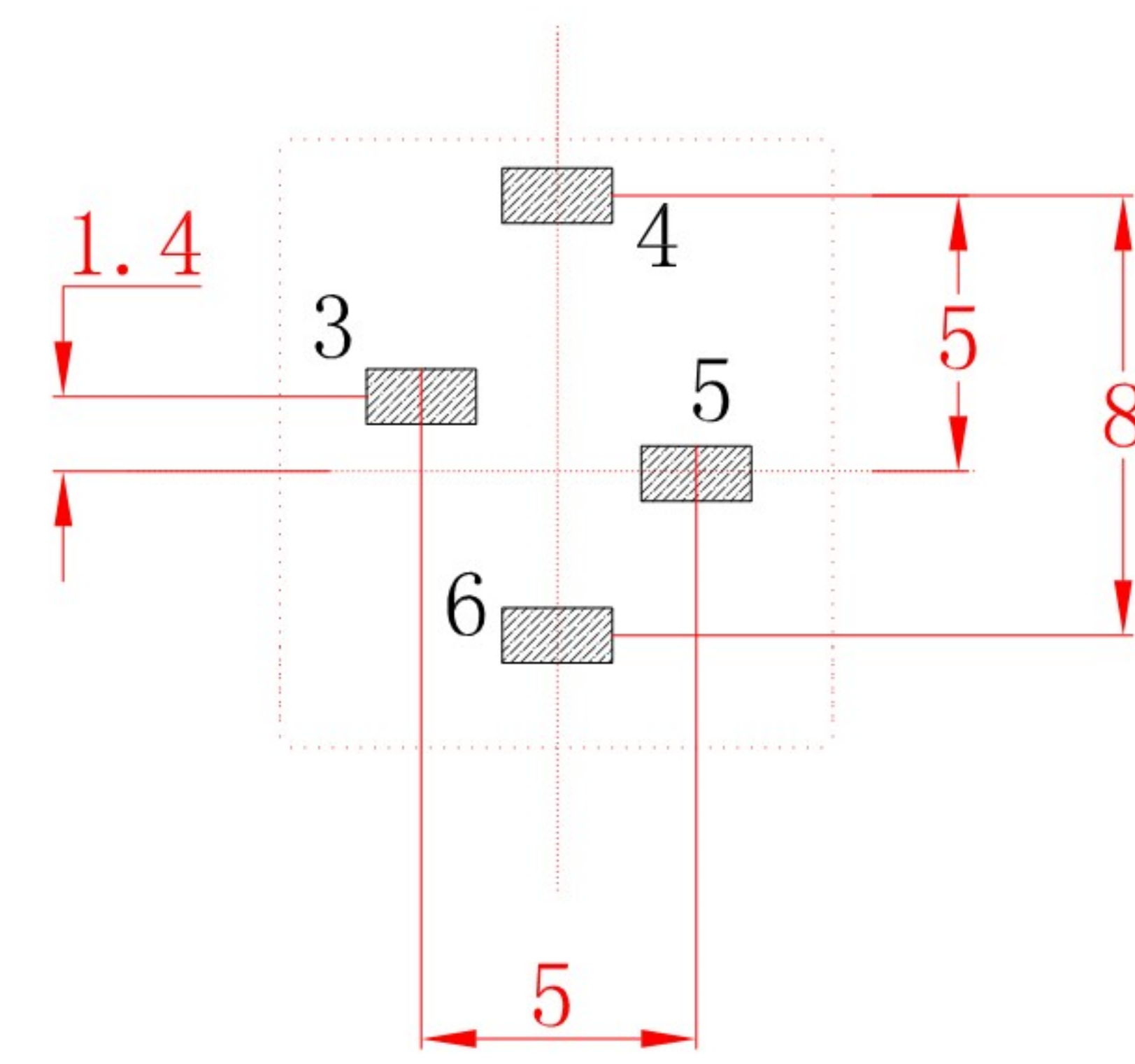
线路板开孔尺寸
