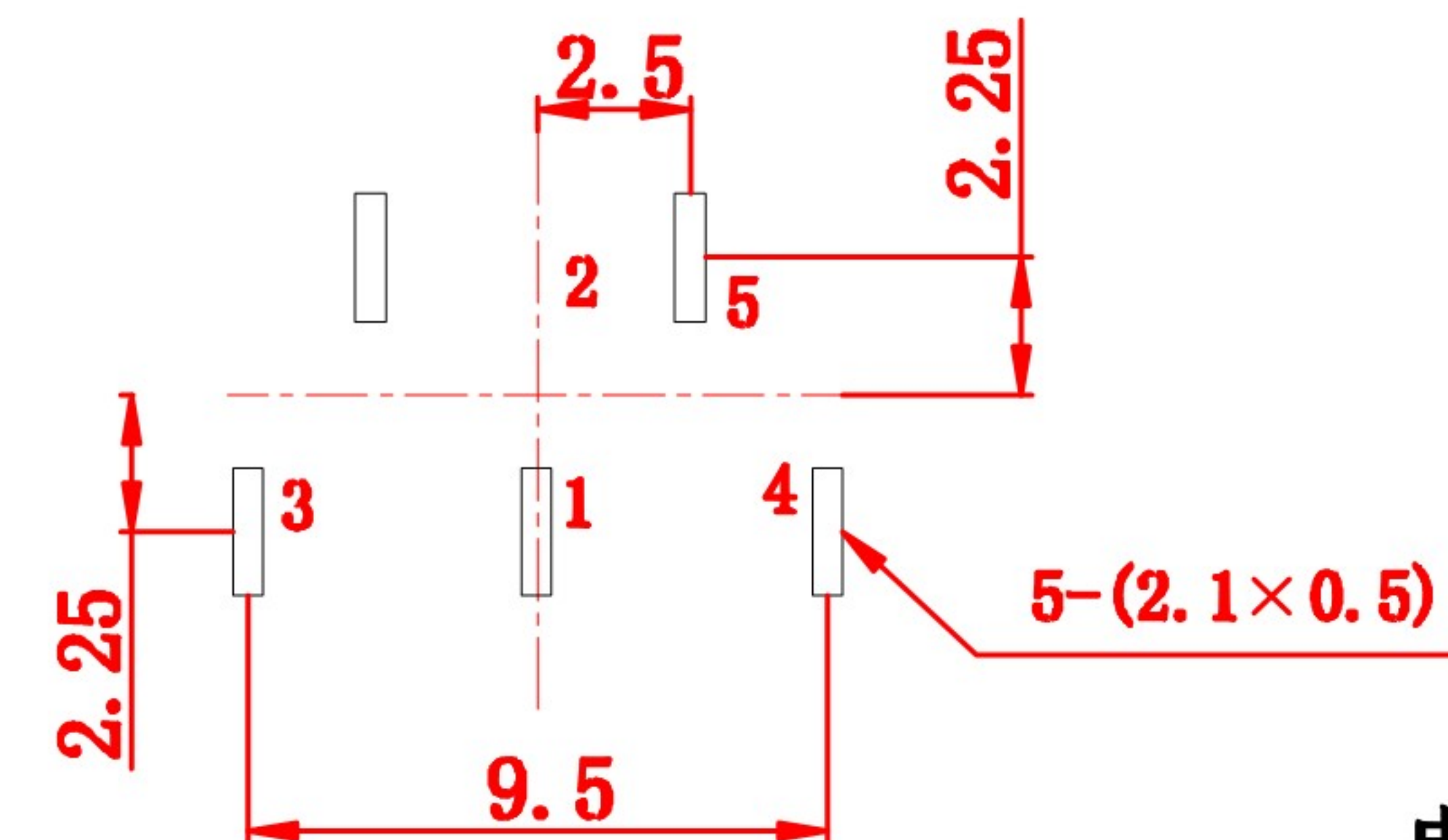
线路板开孔尺寸
