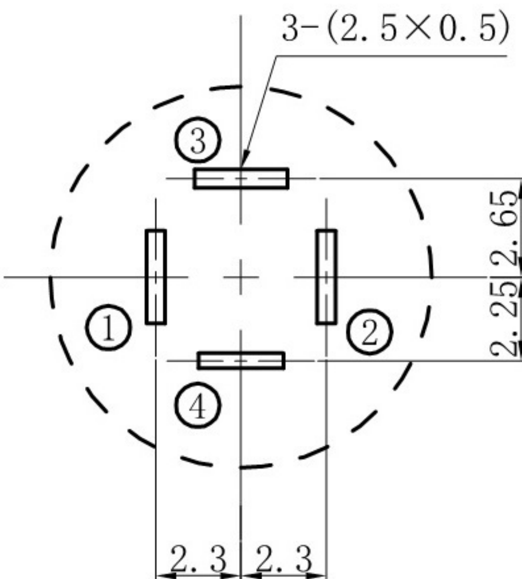
推荐PCB板开孔尺寸
