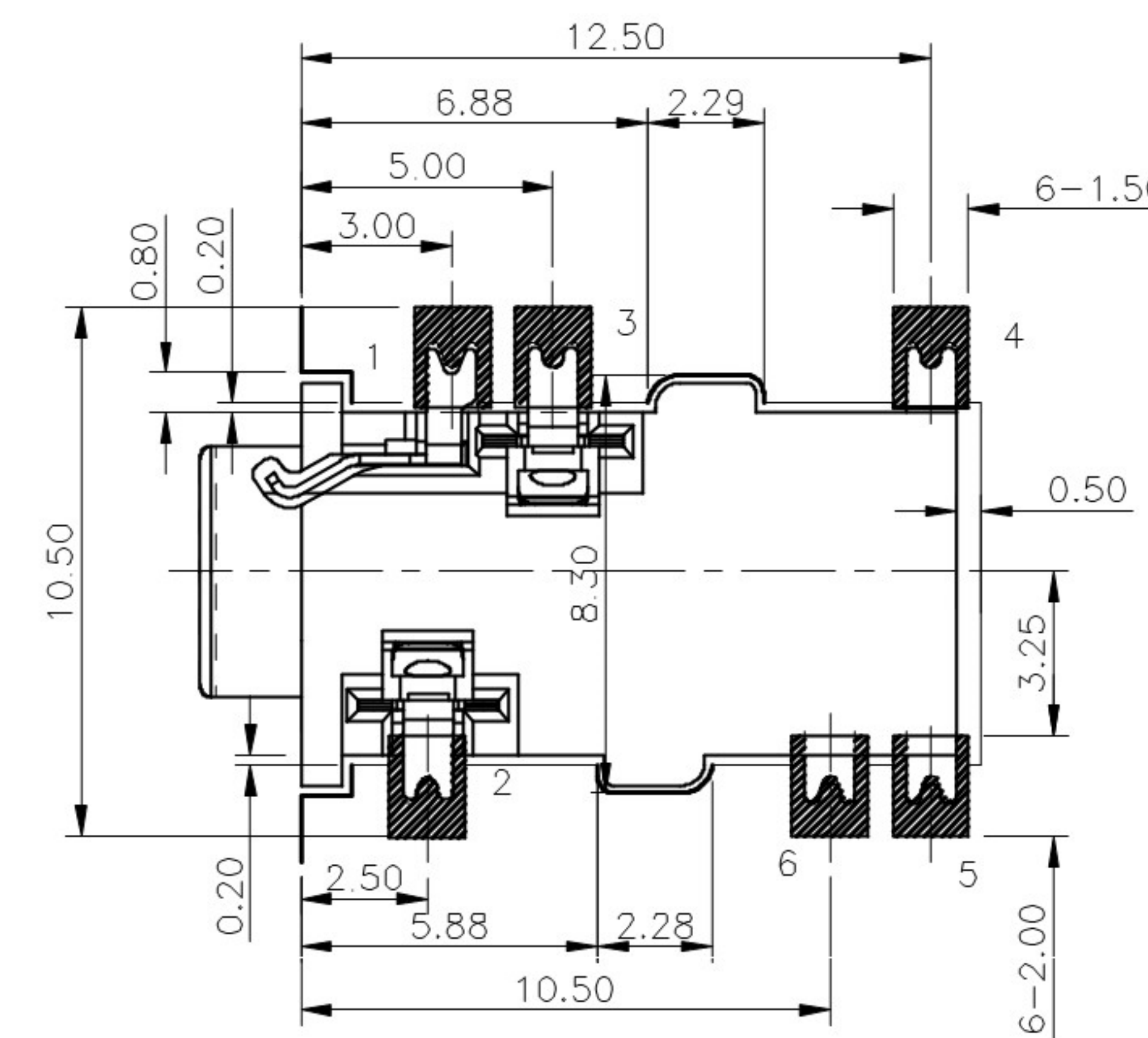
P.C.B LAYOUT TOP VIEW(REVERSE)
