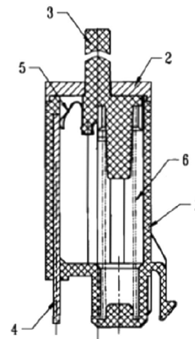
內部構造圖
