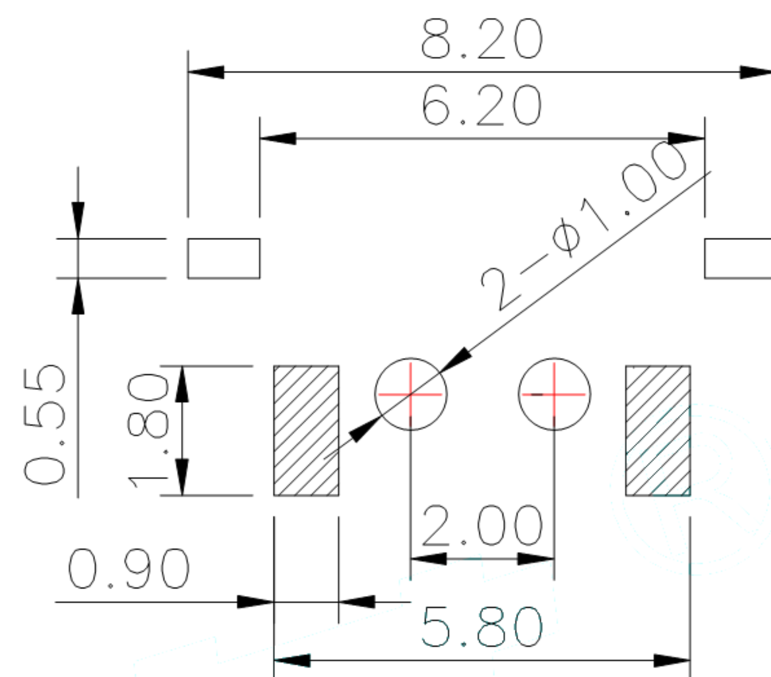
PCB Layout(Pattern side)
