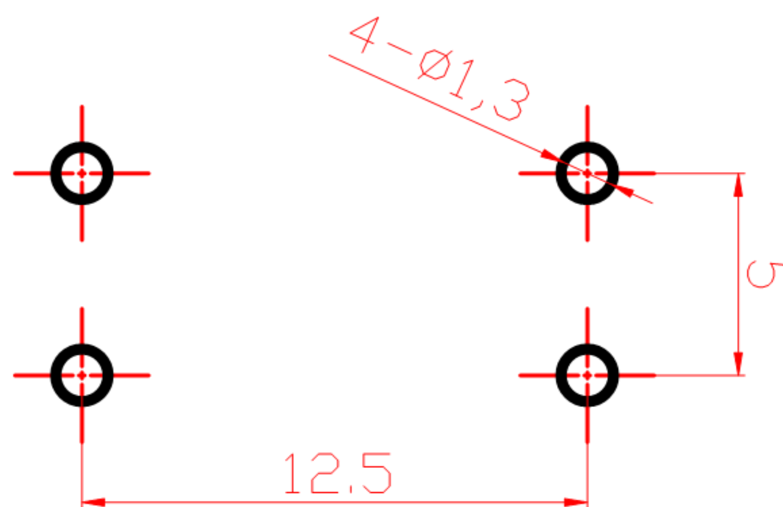
PCB. 焊接图
