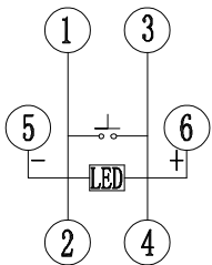
电原理图
