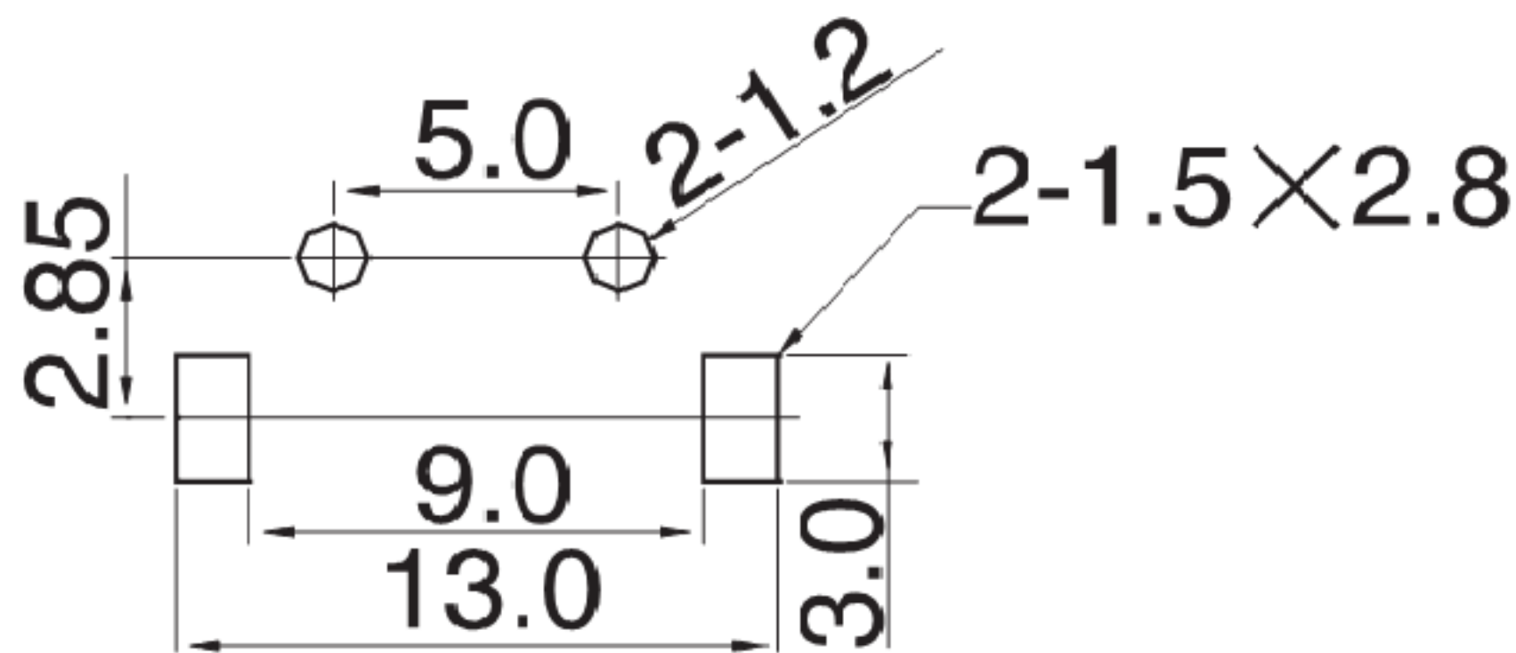
P.C.B.Land Pattern
