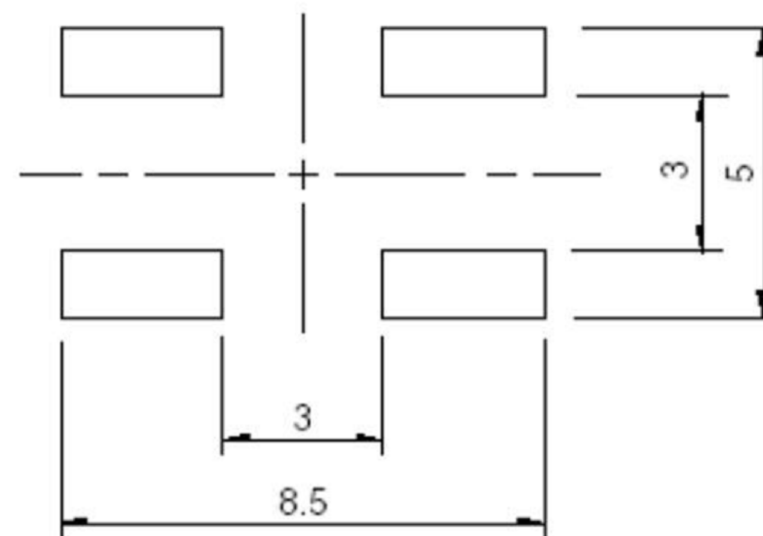
PCB封装
