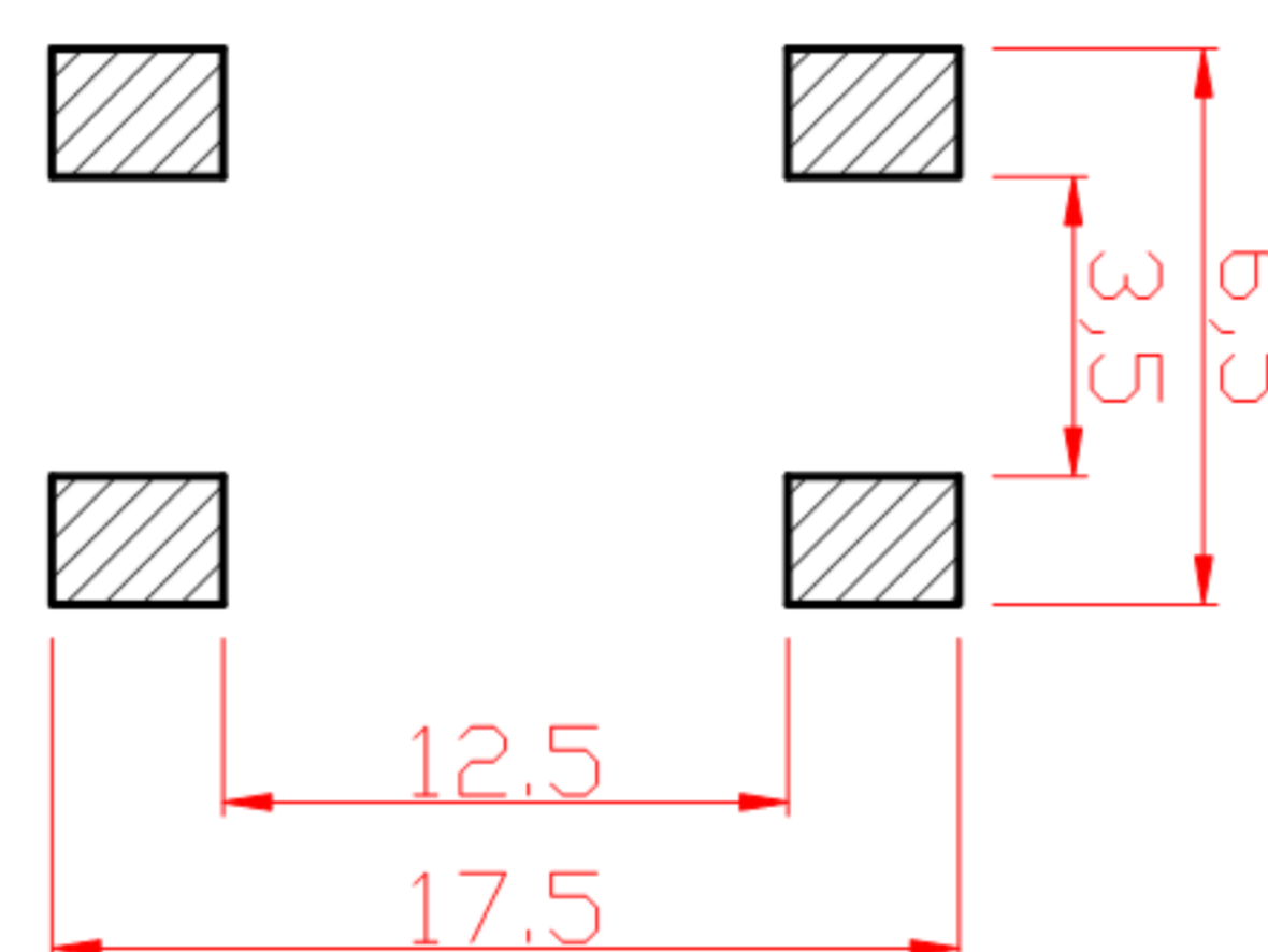
PCB. 焊接图
