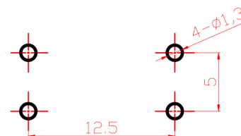
PCB. 焊接图
