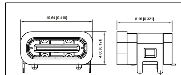
带防水圈示意图
