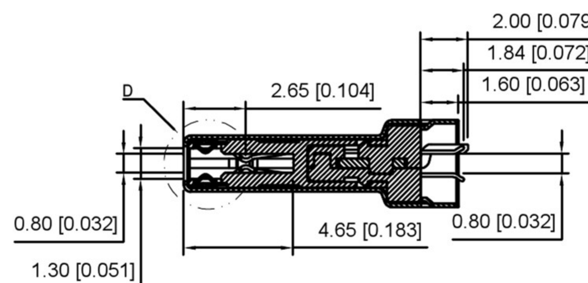
SECT A-A
