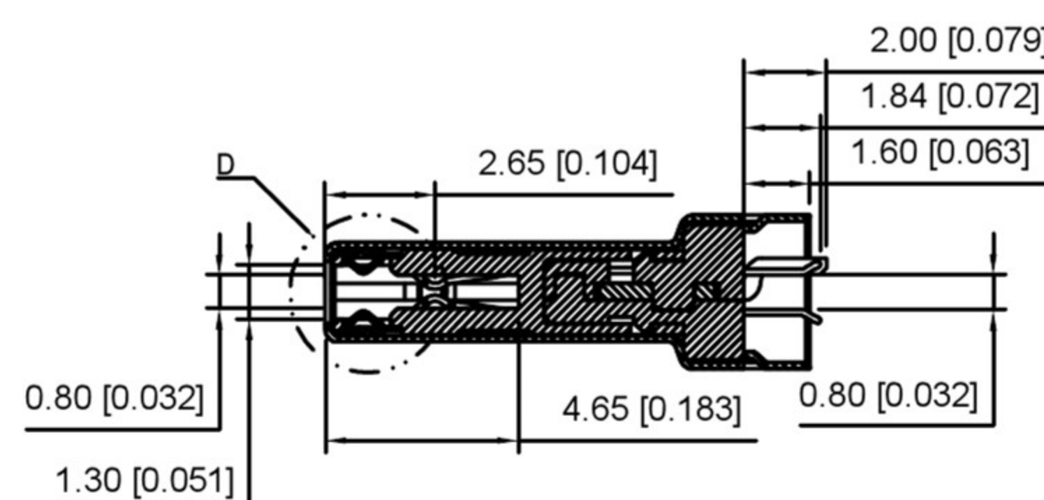
SECT A-A
