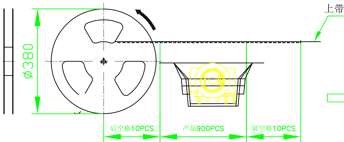
① 产品装入载带
