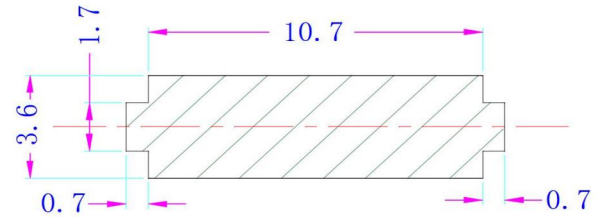
PCB板开孔尺寸
