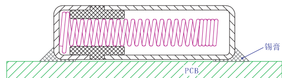
PCB 贴板焊接
