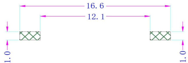
PCB板焊接尺寸
