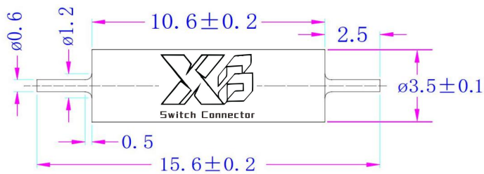
正面图
