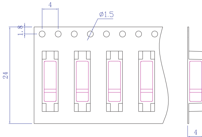
编带示意图
