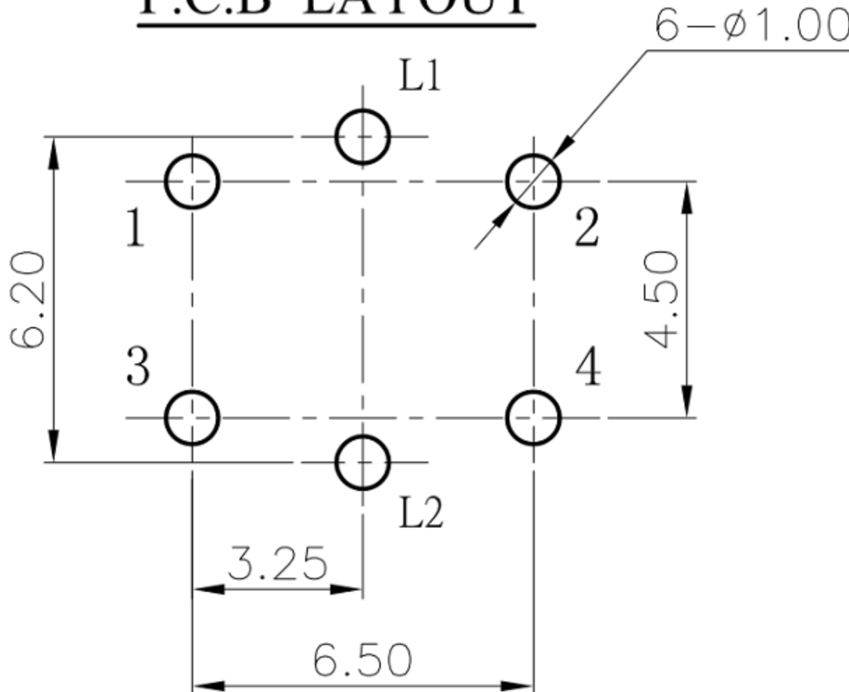
P.C.B LAYOUT
