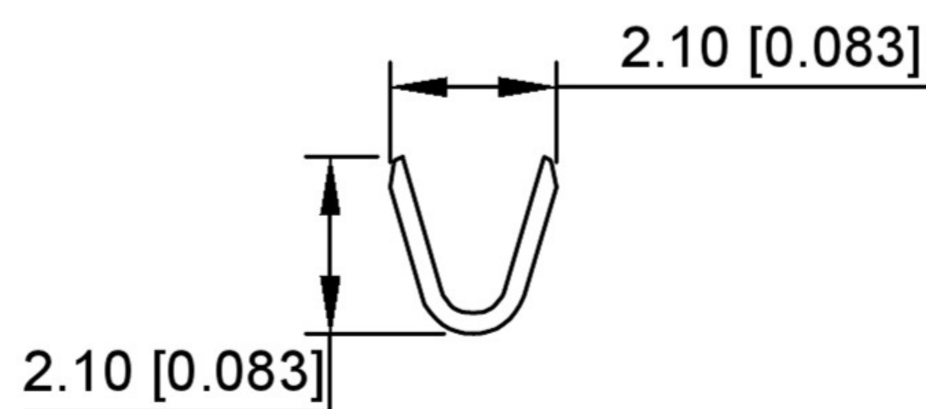
SEC:B-B
