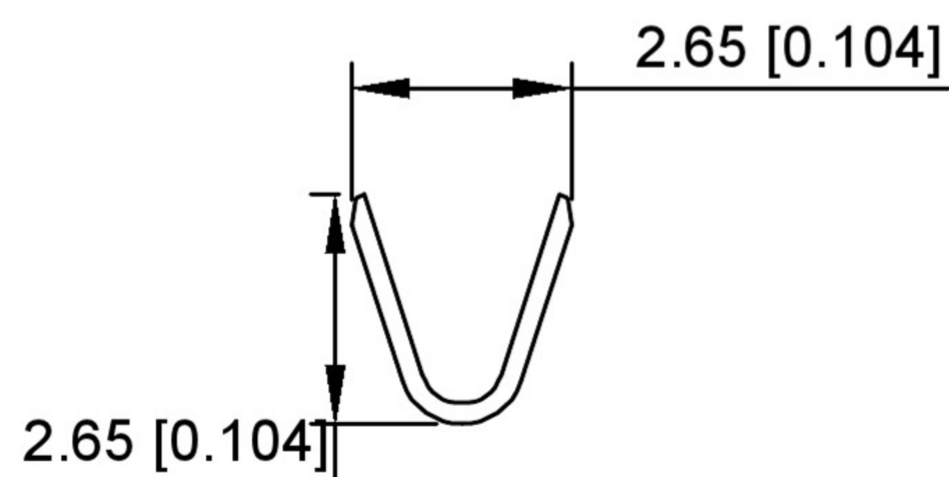
SEC:A-A
