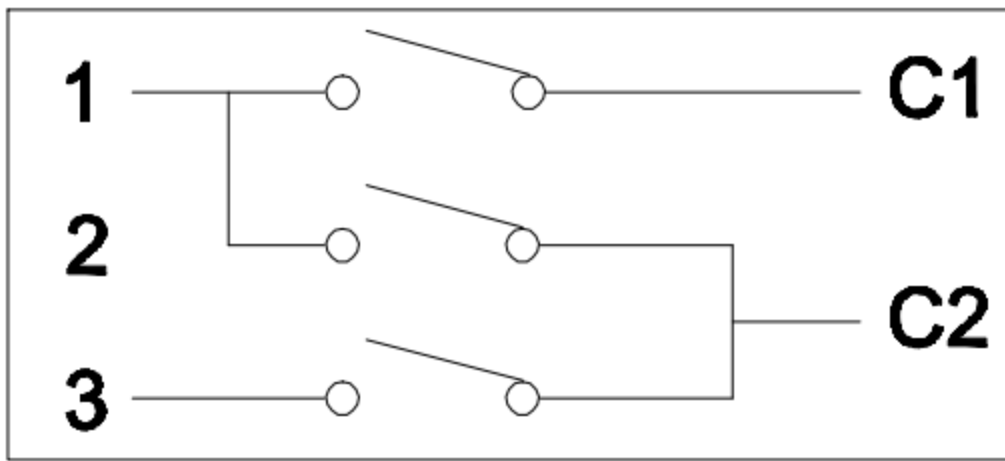
线路图 CIRCUIT DIAGRAM
