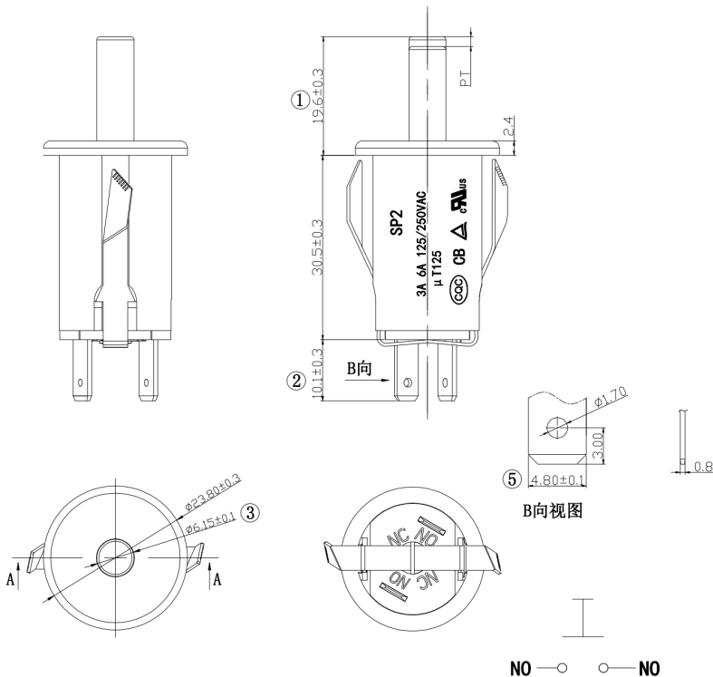
电路图/Circuit diagram
