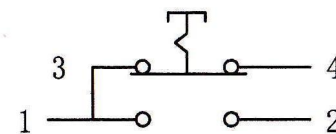
电原理图 CIRCUIT DIAGRAM
