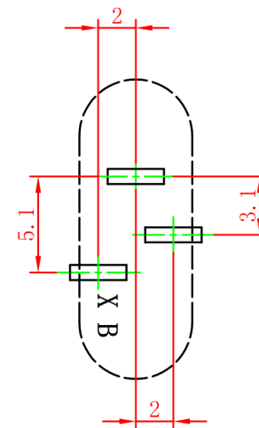
线路板安装尺寸示意图
