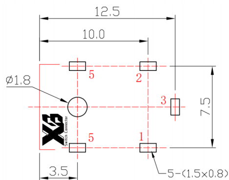
PCB尺寸图
