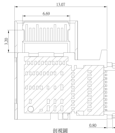
剖視圖
