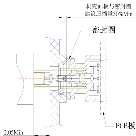
組裝面板後公母頭對插示意圖
