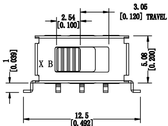
ACTUATOR IN POS. 1
