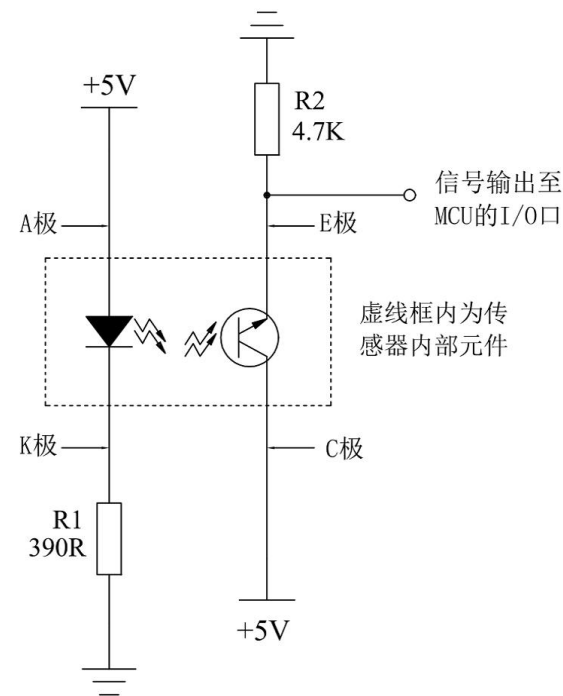
传感器内部电路元件与外部引脚连接图 R1与R2为外接电阻
