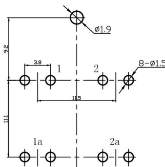
印制板开孔尺寸(±0.1mm)
