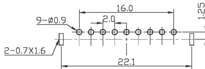
P.C.B. LAYOUT
