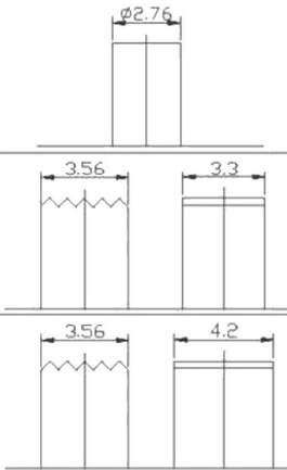
OPTIONAL KNOB TYPE
