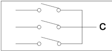
线路图 CIRCUIT DIAGRAM
