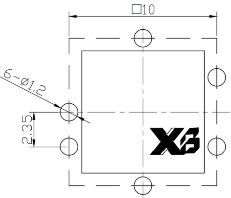
PCB板位置图
