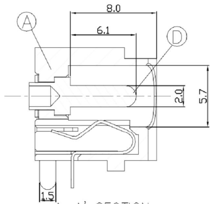
A-A' SECTION
