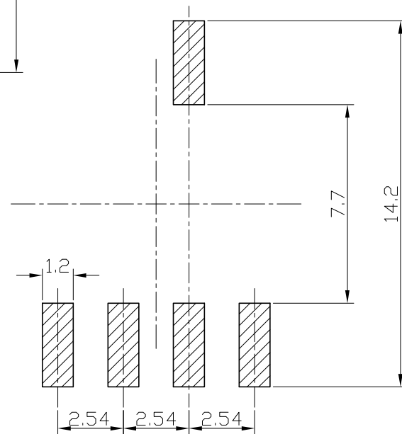
P.C.B LAYOUT
