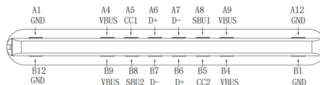
接点定义放大图 (16P)
