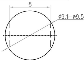
取付穴参考寸法 Mounting hole dimension
