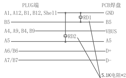
线路原理图
