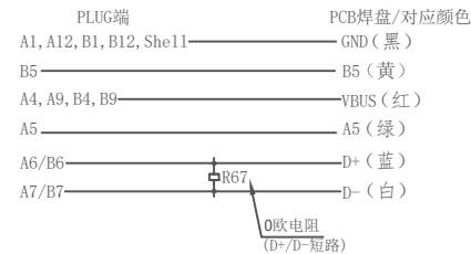
线路原理图
