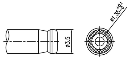
DC PLUG-REF
