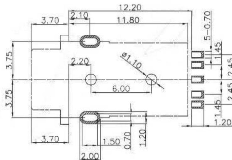
P.C.B Layout
