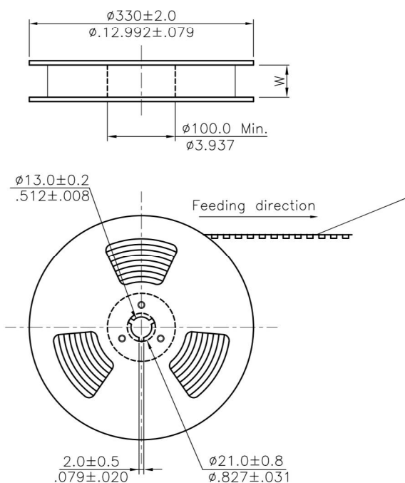
REEL DIMENSIONS
